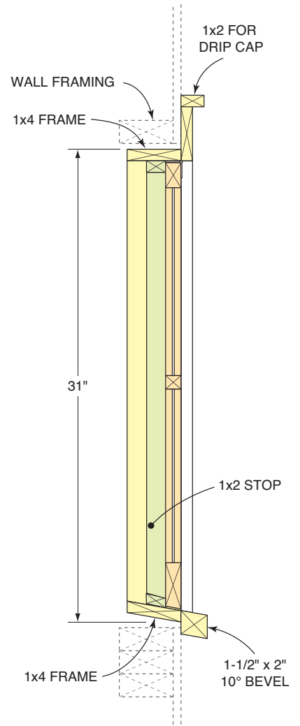
SECTION A-A
